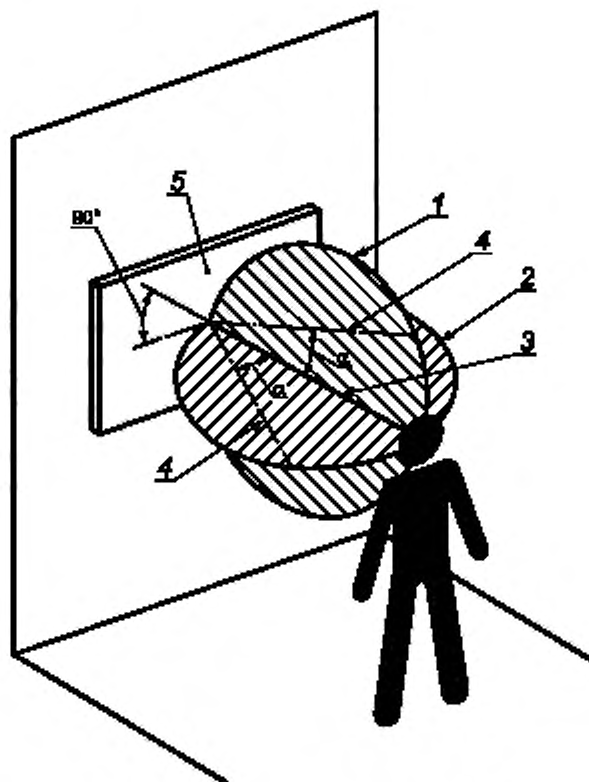
Рисунок А.2 — Вертикальные и горизонтальные плоскости для расстояния распознавания одинаковой идентифицируемости элементов графических символов знака безопасности
